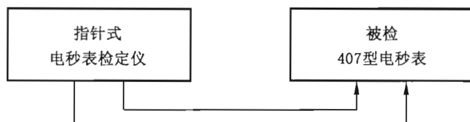
图 3 407 型电秒表的检定
